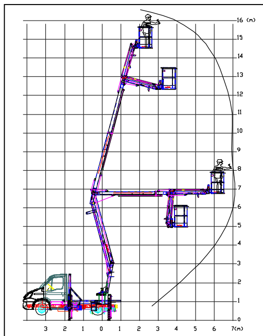
Pracovní diagram
