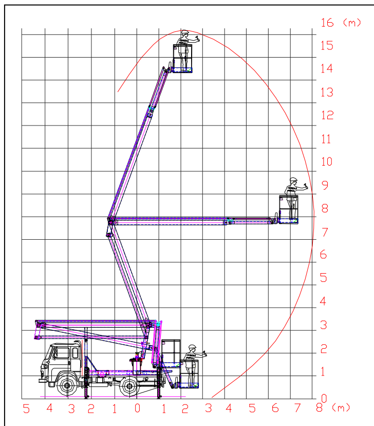
Pracovní diagram
