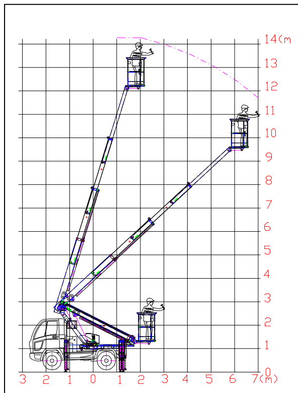
Pracovní diagram
