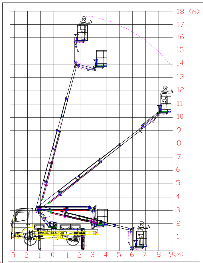
Pracovní diagram
